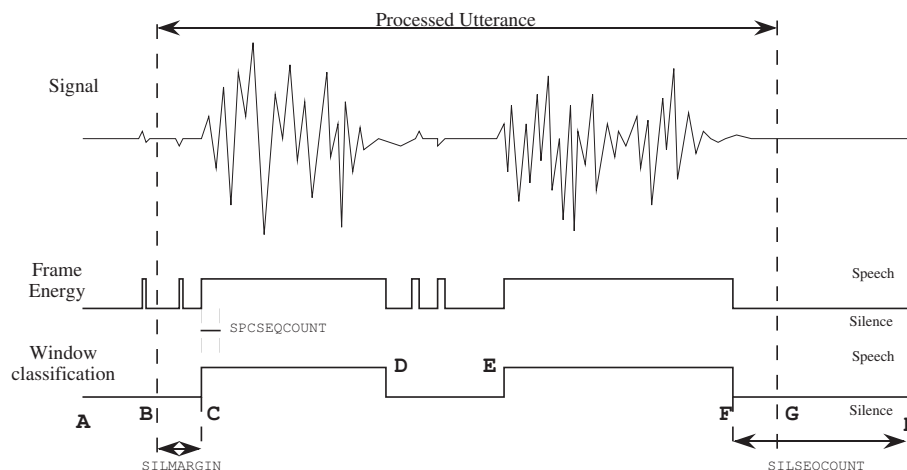
Fig. 5.6 Endpointer Parameters
